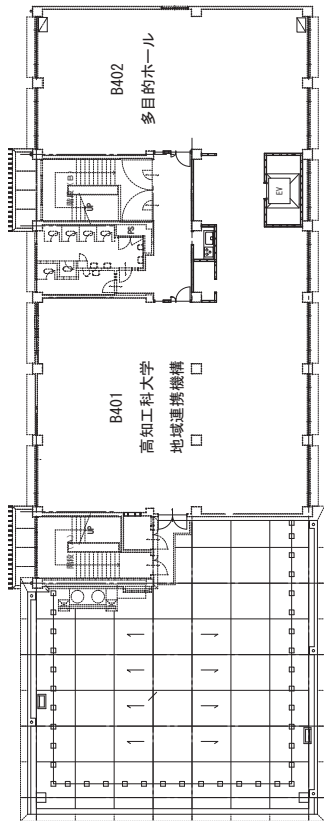
4 階平面図
