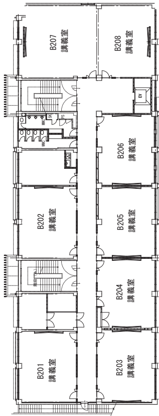
2階平面図
