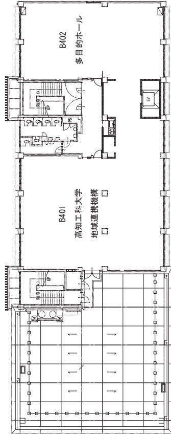
4階平面図
