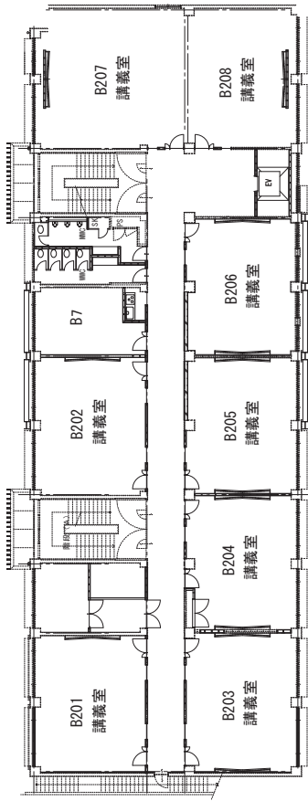
2階平面図
