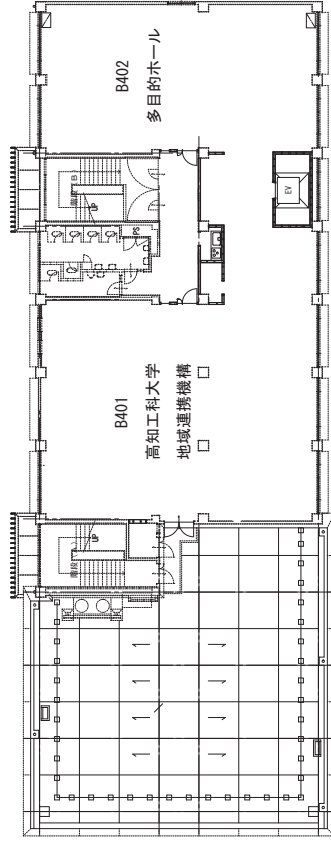
4階平面図
