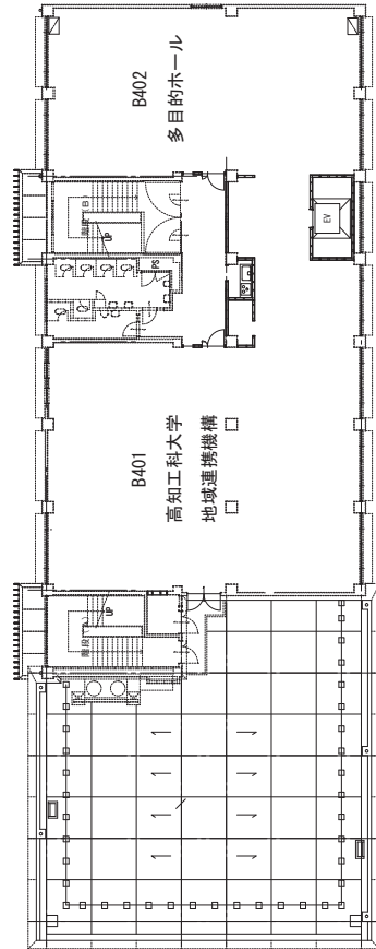
4階平面図
