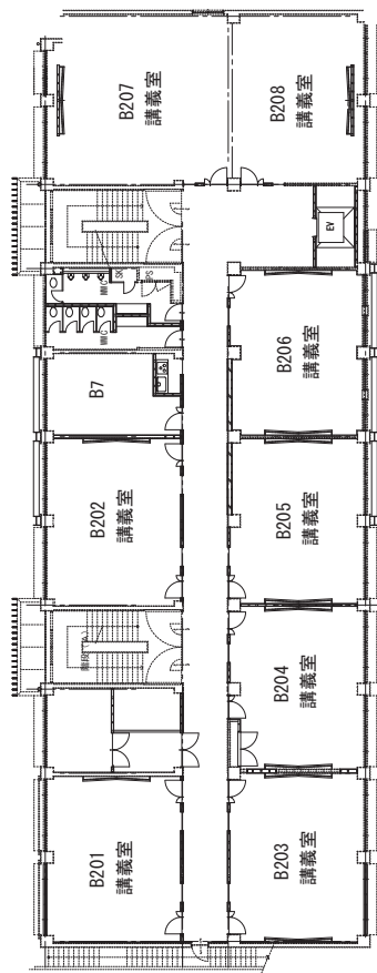
2階平面図
